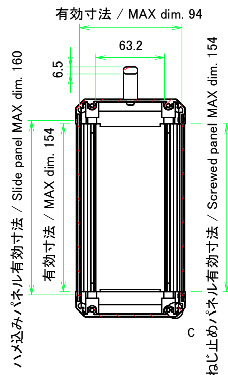
B-B (1 : 3.5)
