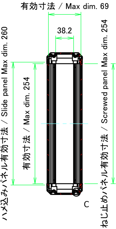
B-B ( 1 : 5 )
