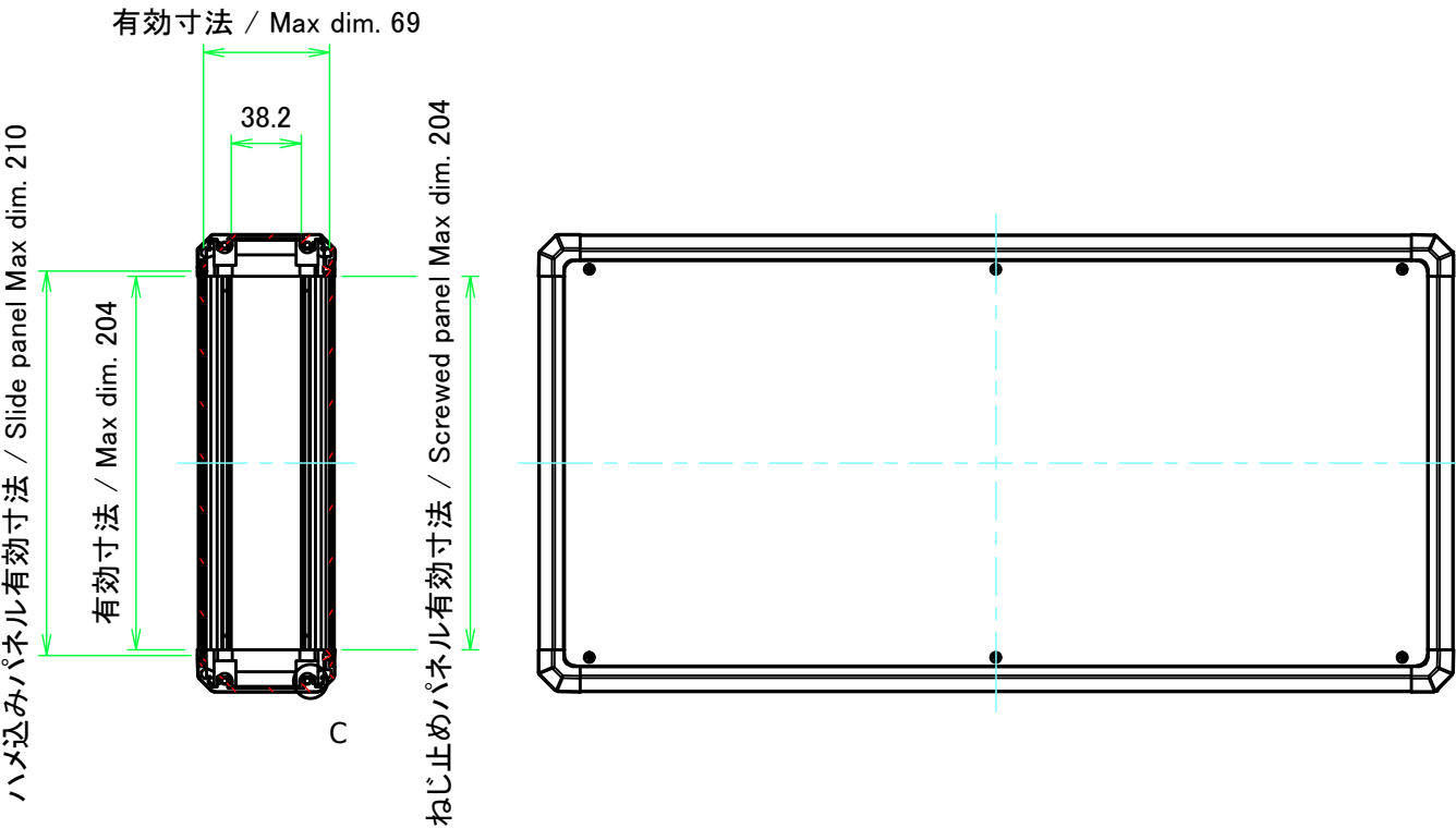
B-B ( 1 : 4.5 )
