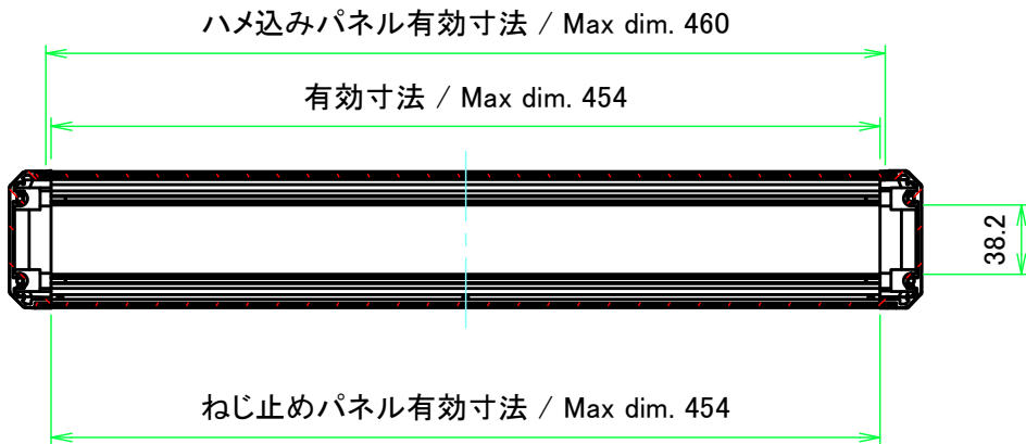
A-A ( 1 : 4.5 )
