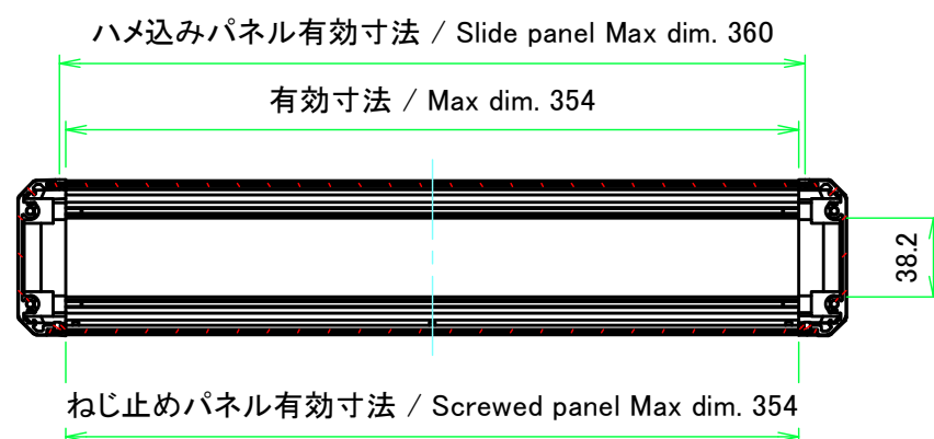
A-A ( 1 : 4 )
