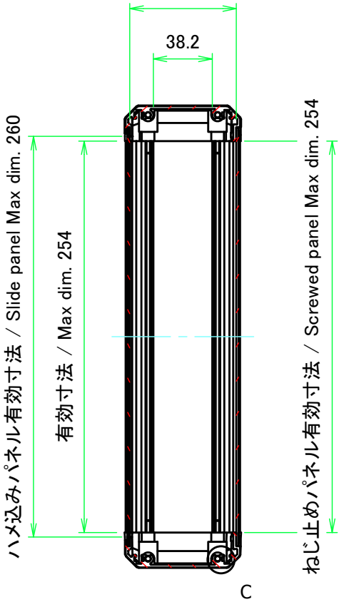
B-B ( 1 : 3.5 )
