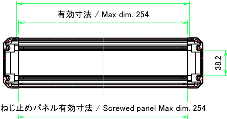
ハメ込みパネル有効寸法 / Slide panel Max dim. 260
