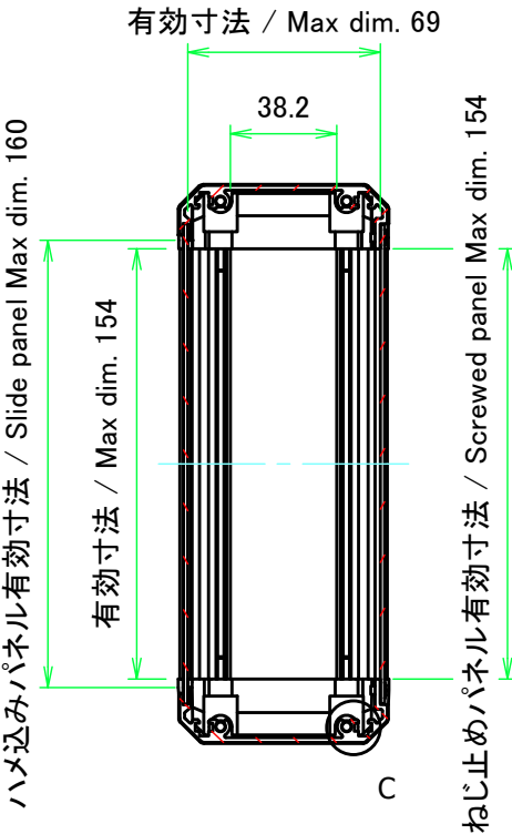
B-B ( 1 : 3 )
