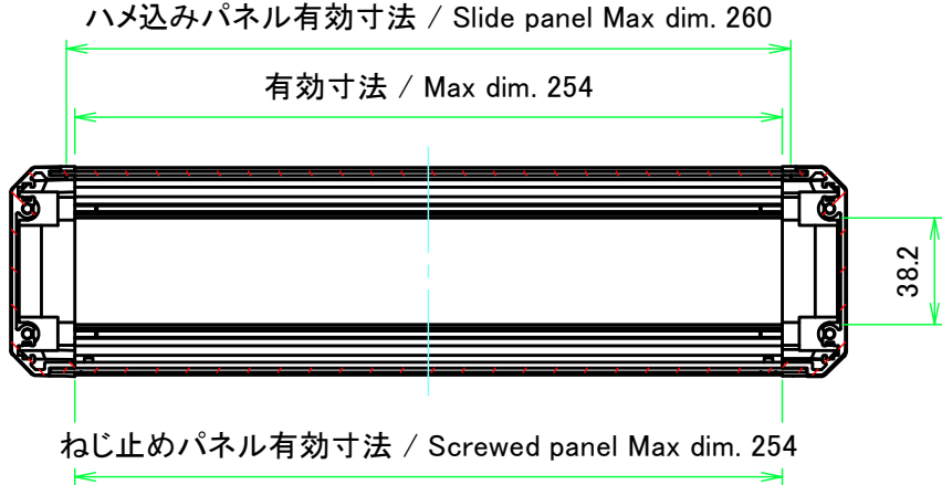
A-A ( 1 : 3 )
