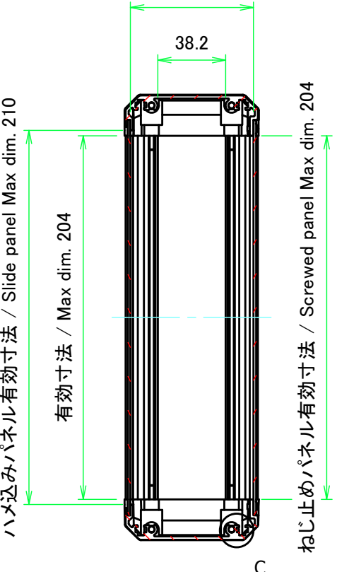
B-B ( 1 : 3 )
