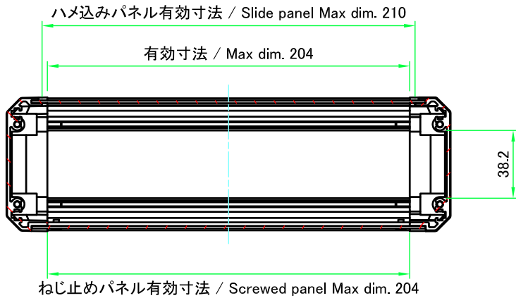
A-A ( 1 : 3 )
