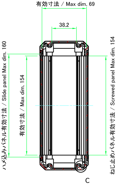
B-B ( 1 : 3 )
