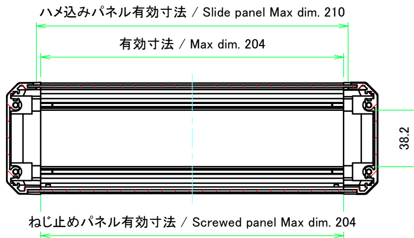
A-A ( 1 : 2.5 )
