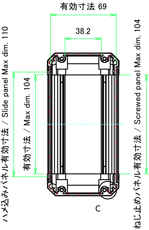
B-B ( 1 : 2.5 )
