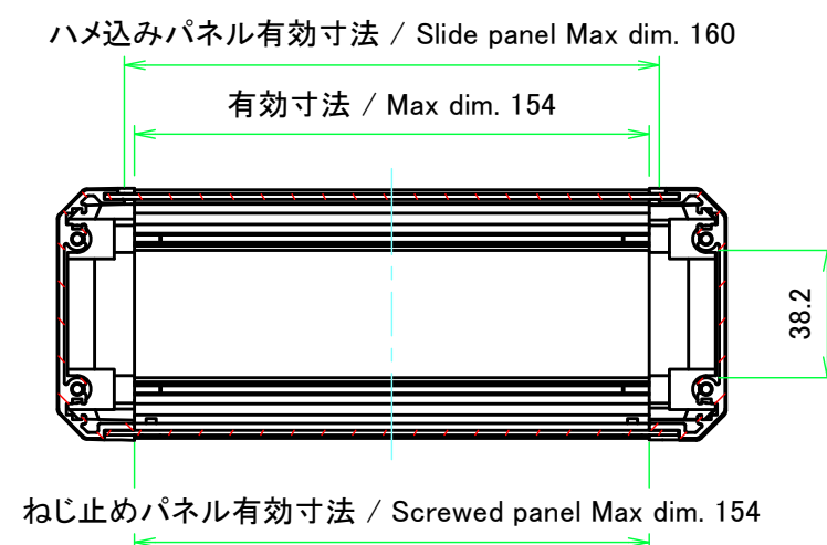
A-A ( 1 : 2.5 )
