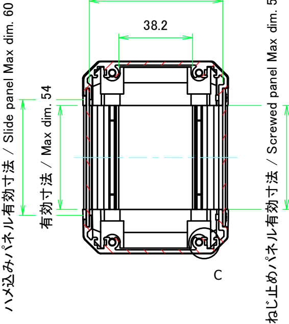
C : フレーム拡大図 / Frame cross-section
