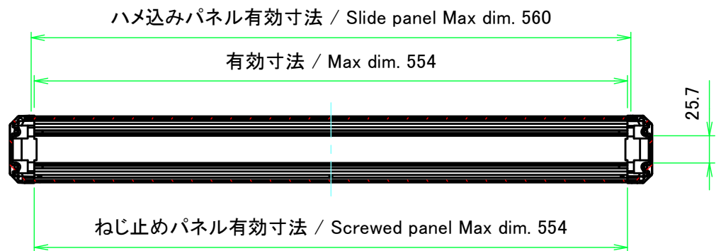
A-A ( 1 : 5 )
