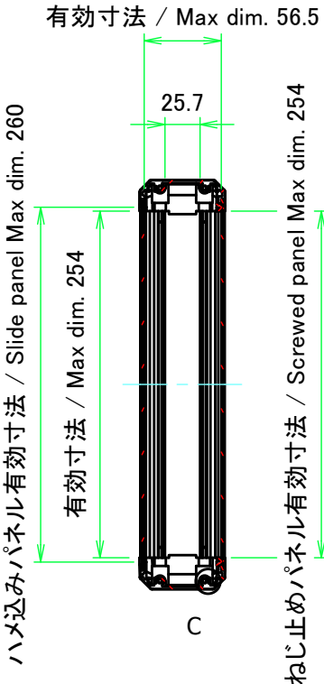
フレーム4側 / Frame4 side
