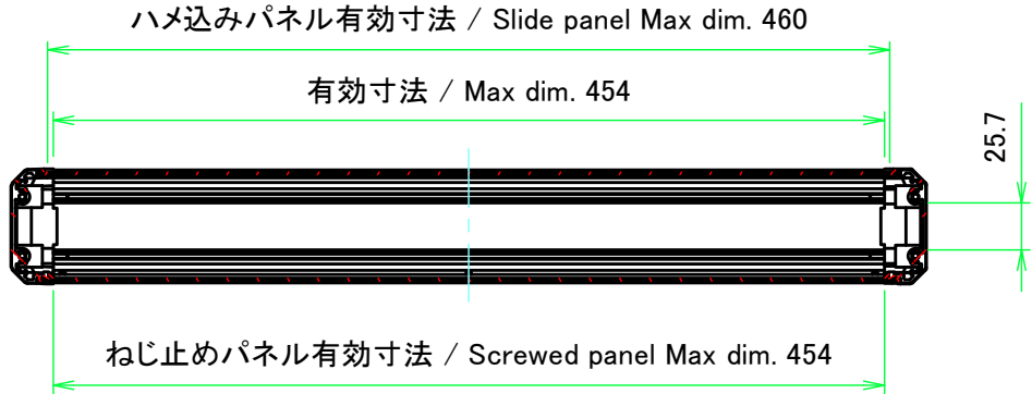
A-A ( 1 : 4.5 )
