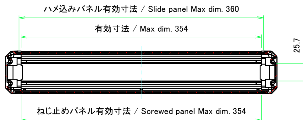
A-A ( 1 : 3.5 )
