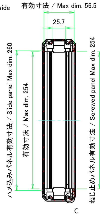
B-B ( 1 : 3.5 )
