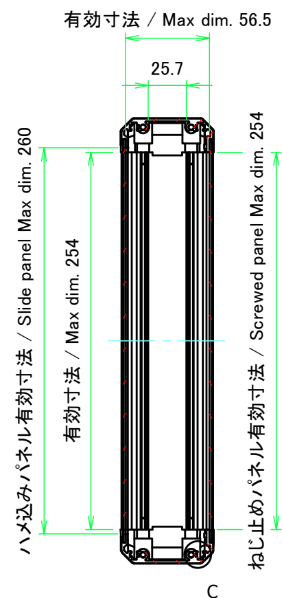
B-B ( 1 : 3.5 )
