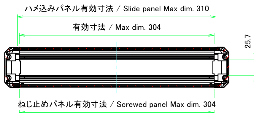
A-A ( 1 : 3.5 )
