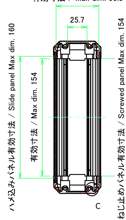
B-B ( 1 : 3 )
