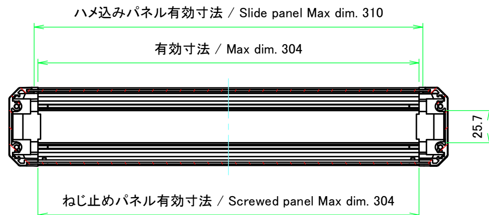
A-A ( 1 : 3 )
