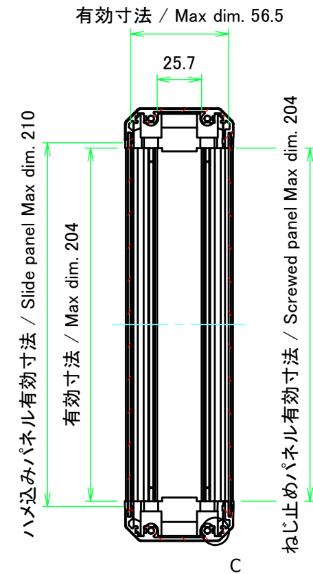
B-B ( 1 : 3 )
