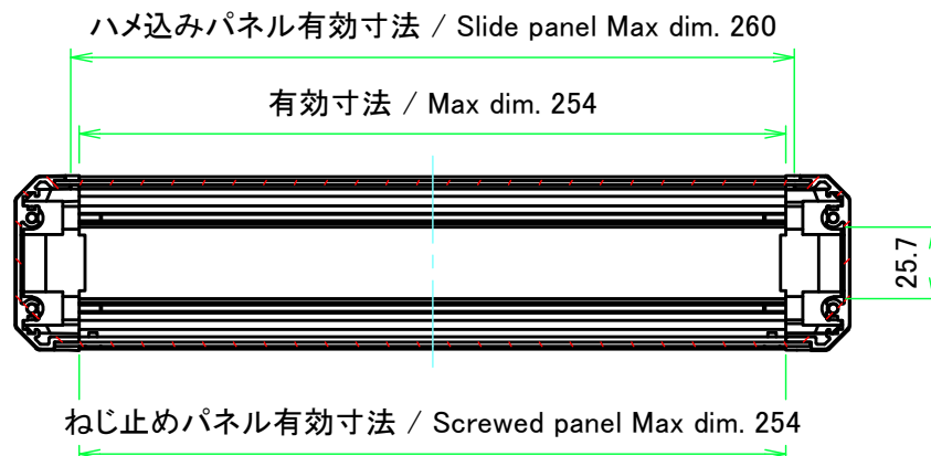
A-A ( 1 : 3 )
