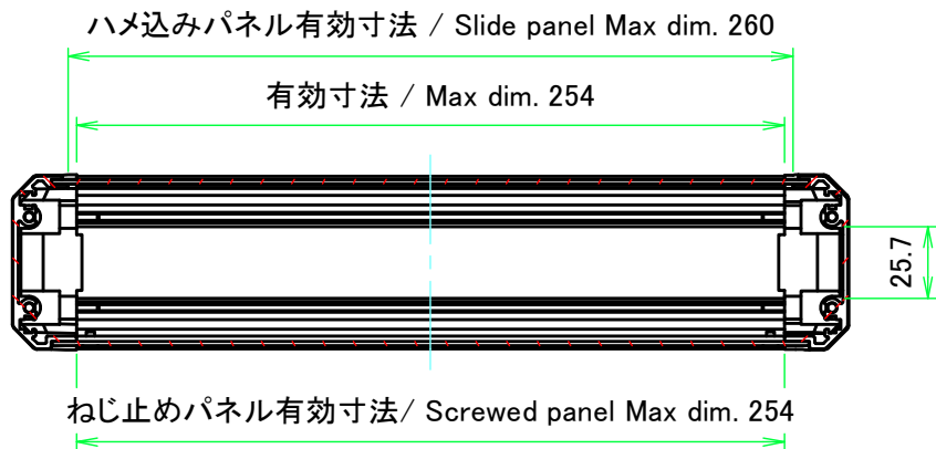
A-A ( 1 : 3 )
