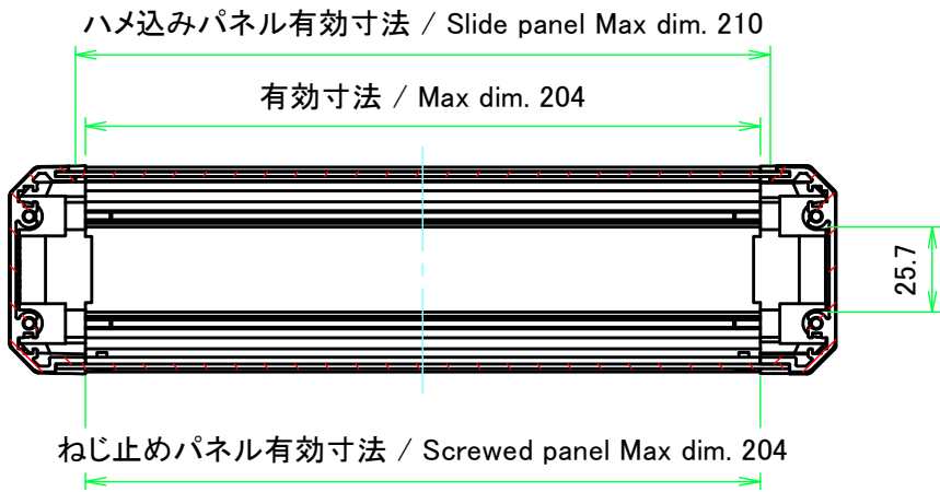
A-A ( 1 : 2.5 )
