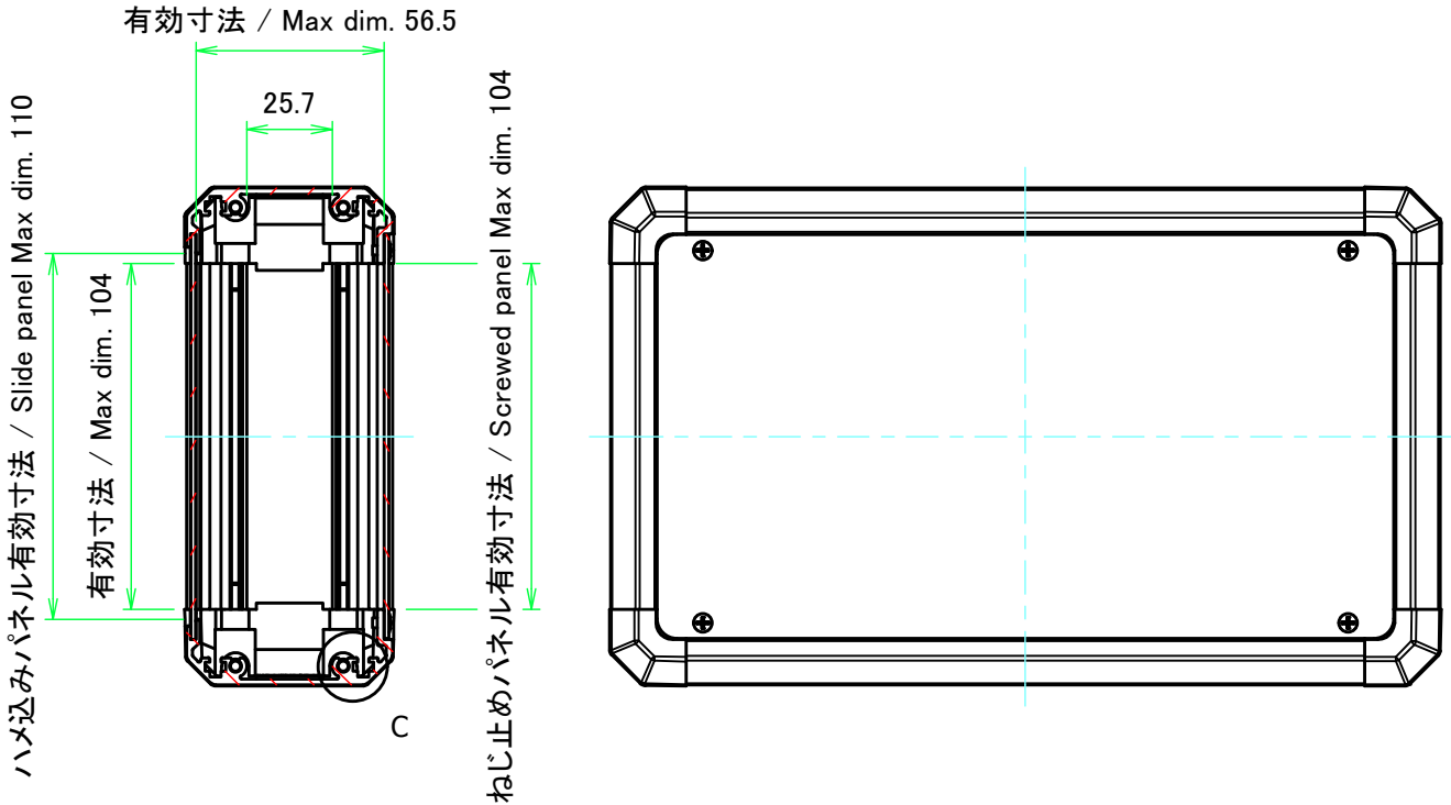
B-B ( 1 : 2.5 )
