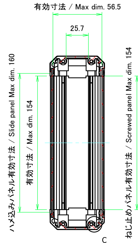
B-B ( 1 : 2.5 )
