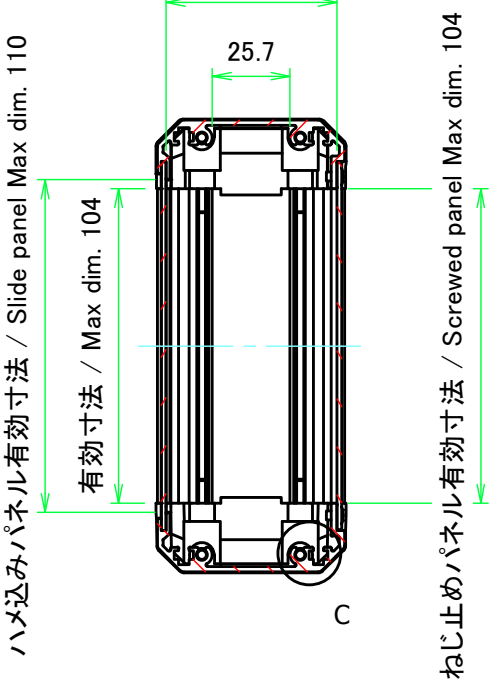
B-B ( 1 : 2.5 )
