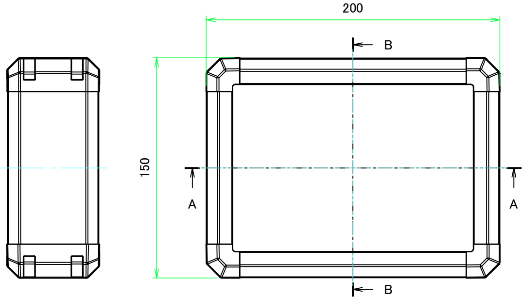
フレーム3側 / Frame3 side
