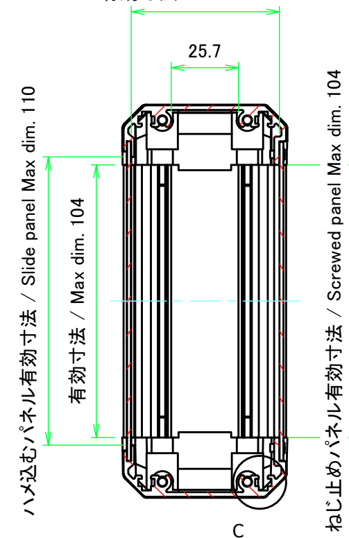
B-B ( 1 : 2 )
