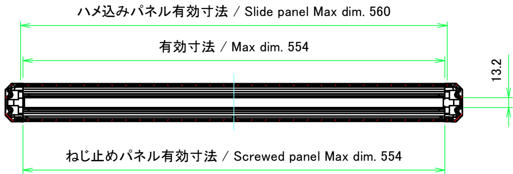
A-A ( 1 : 5 )
