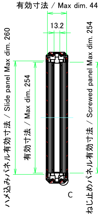
B-B ( 1 : 5 )
