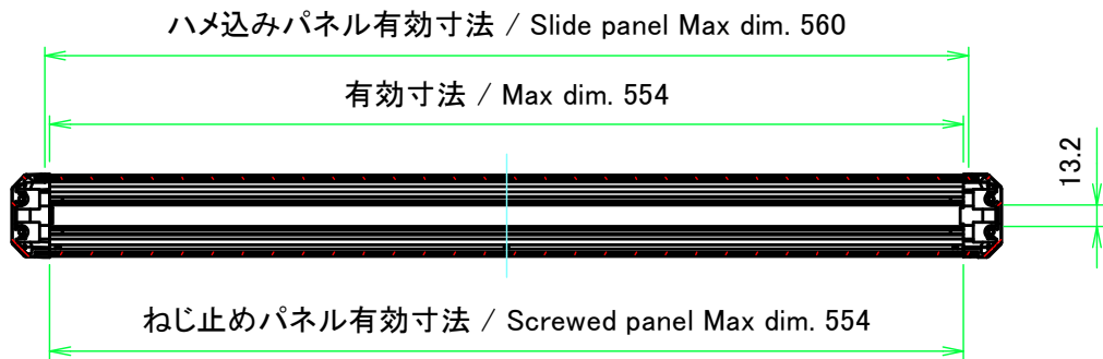
A-A ( 1 : 5 )
