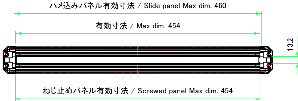
A-A ( 1 : 4 )
