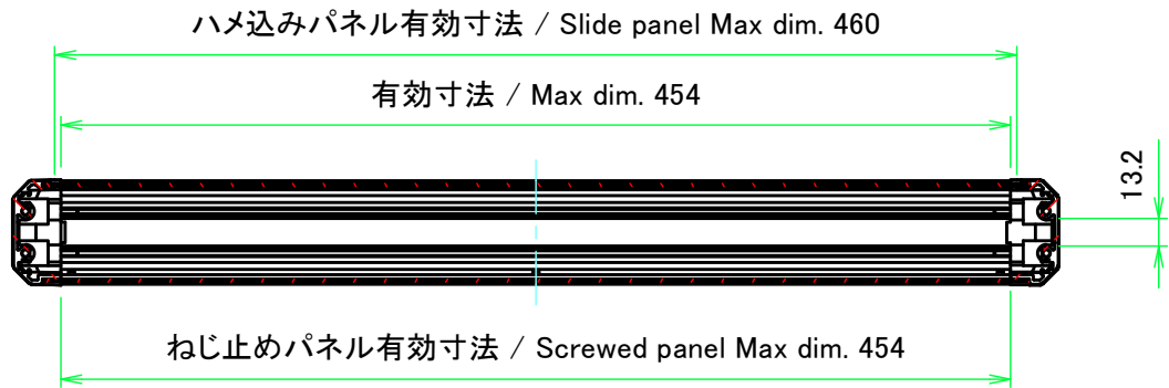
A-A ( 1 : 4 )
