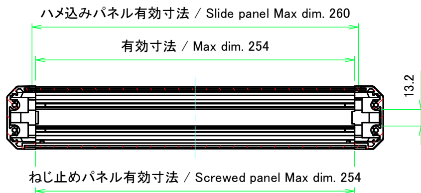
A-A ( 1 : 3 )
