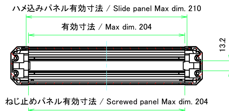
A-A ( 1 : 3 )
