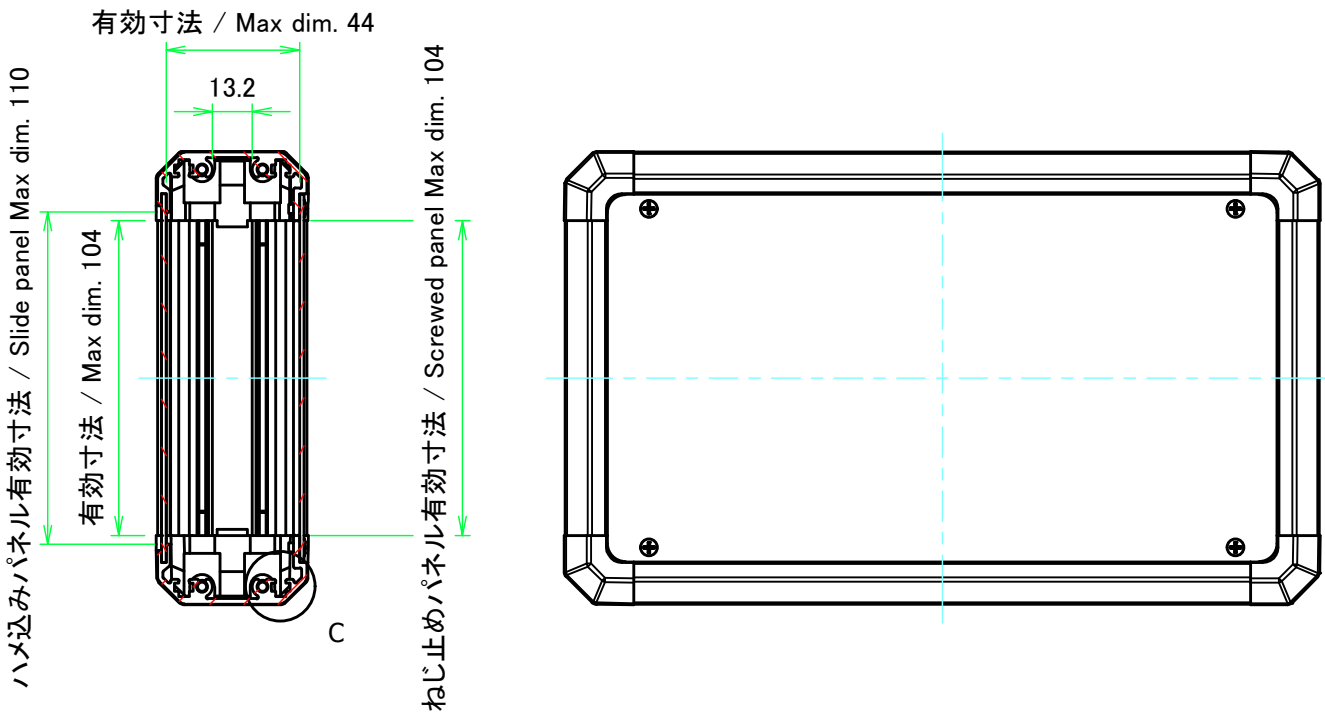
B-B ( 1 : 2.5 )
