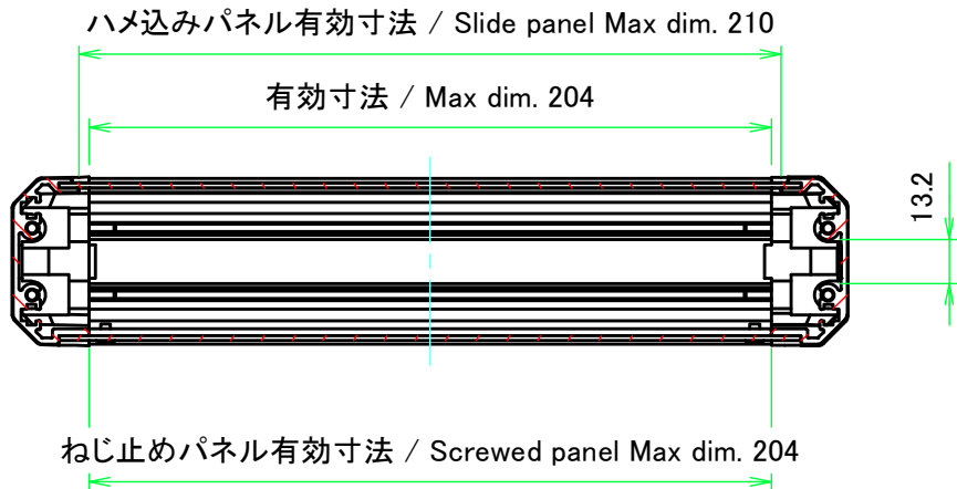
A-A ( 1 : 2.5 )
