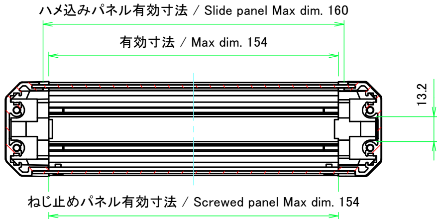
A-A ( 1 : 2 )
