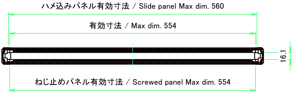
A-A ( 1 : 5 )
