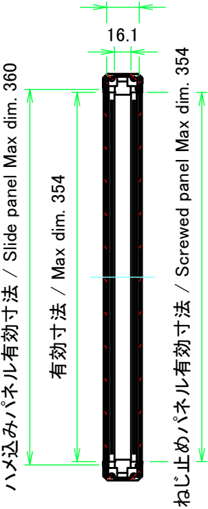
B-B ( 1 : 5 )
