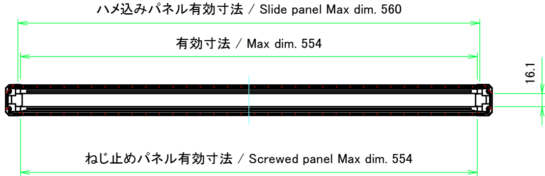
A-A ( 1 : 4.5 )
