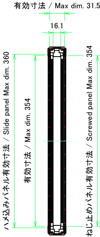
B-B ( 1 : 4.5 )
