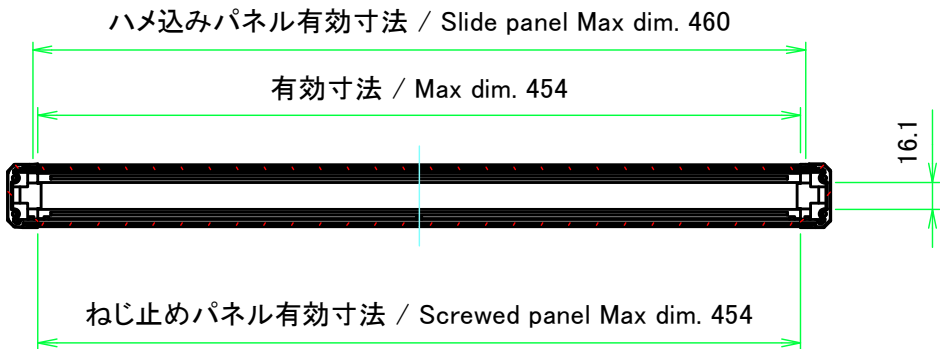
A-A ( 1 : 4.5 )
