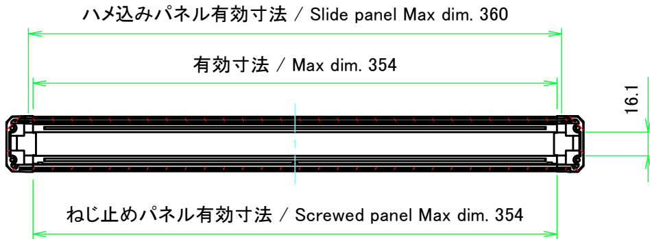
A-A ( 1 : 3.5 )
