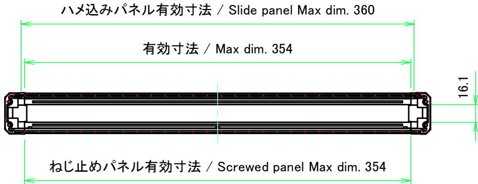
A-A ( 1 : 3.5 )
