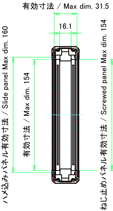
B-B ( 1 : 3 )
