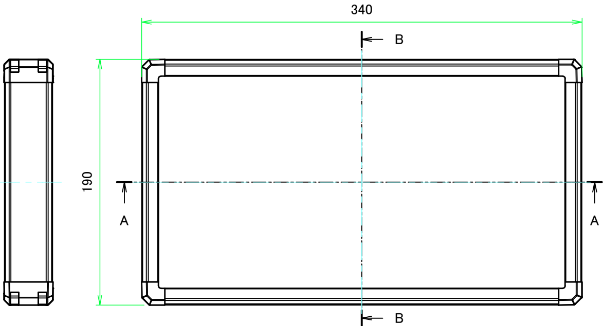
フレーム3側 / Frame3 side
