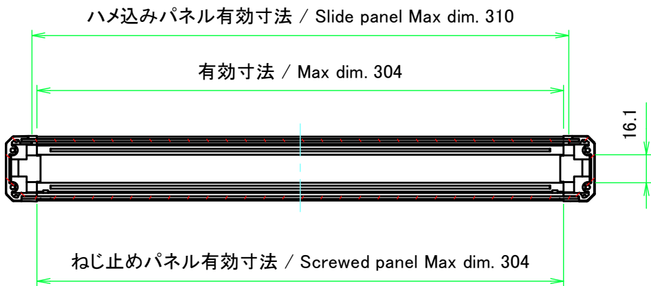
A-A ( 1 : 3 )
