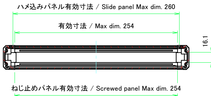
A-A ( 1 : 3 )
