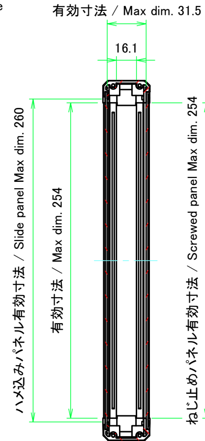
フレーム4側 / Frame4 side
