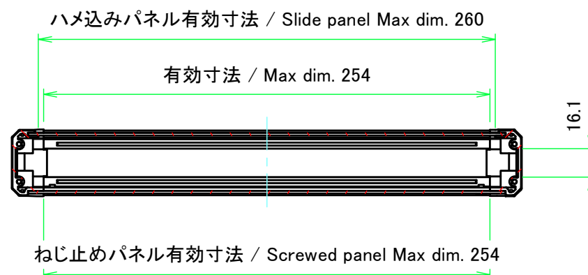
A-A ( 1 : 3 )
