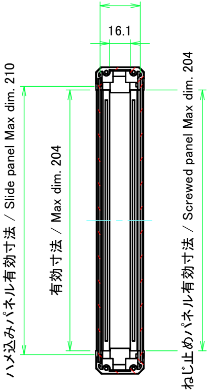
B-B ( 1 : 3 )
