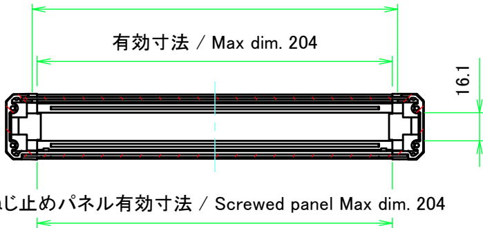
A-A ( 1 : 3 )
