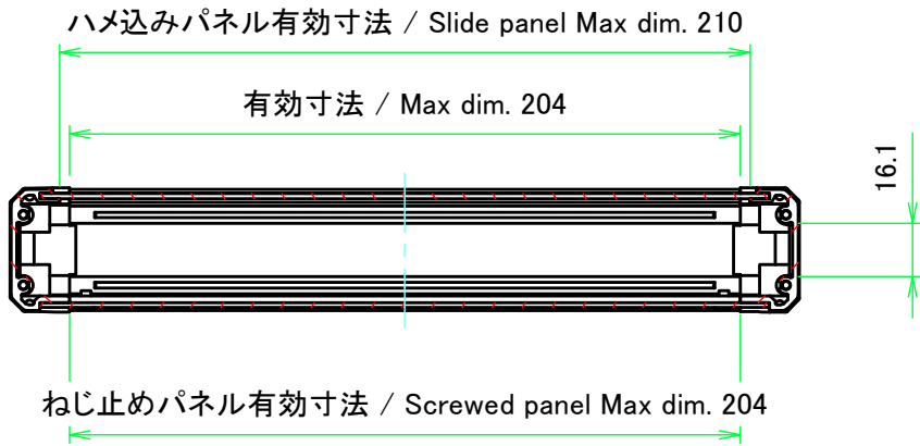
A-A ( 1 : 2.5 )
