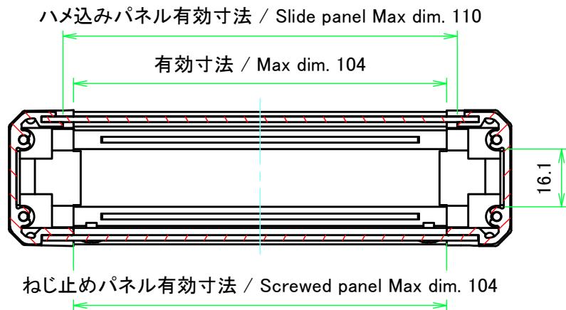
A-A (1:1.5)
