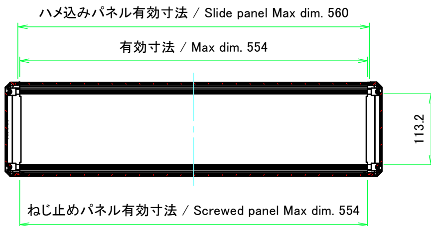
A-A ( 1 : 6 )
