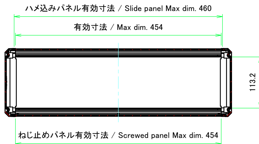
A-A ( 1 : 5 )
