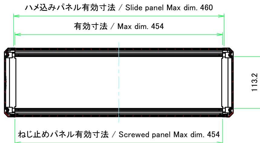
A-A ( 1 : 5 )
