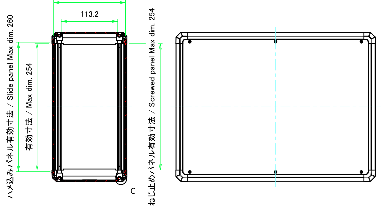
C : フレーム拡大図 / Frame cross-section
