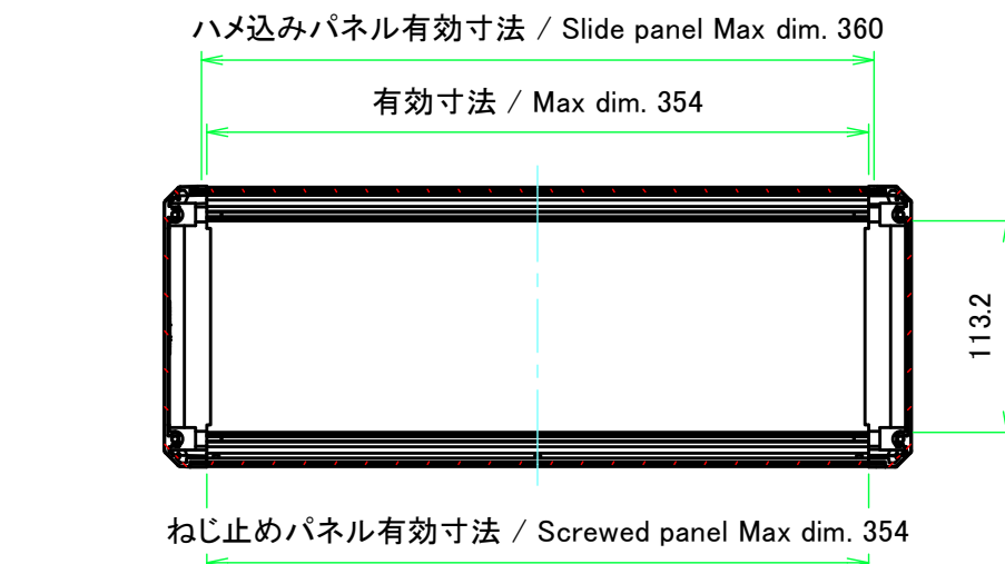
A-A ( 1 : 4.5 )
