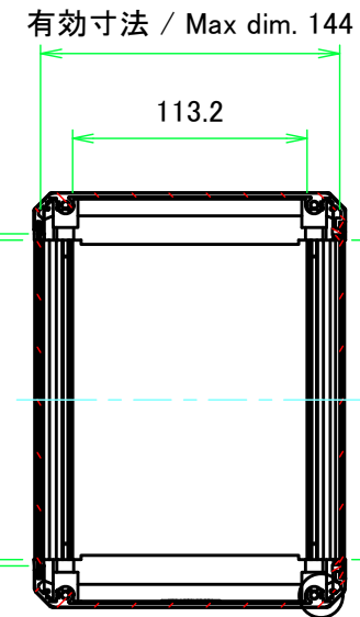
B-B ( 1 : 4 )
