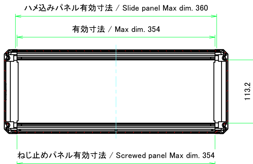
A-A ( 1 : 4 )
