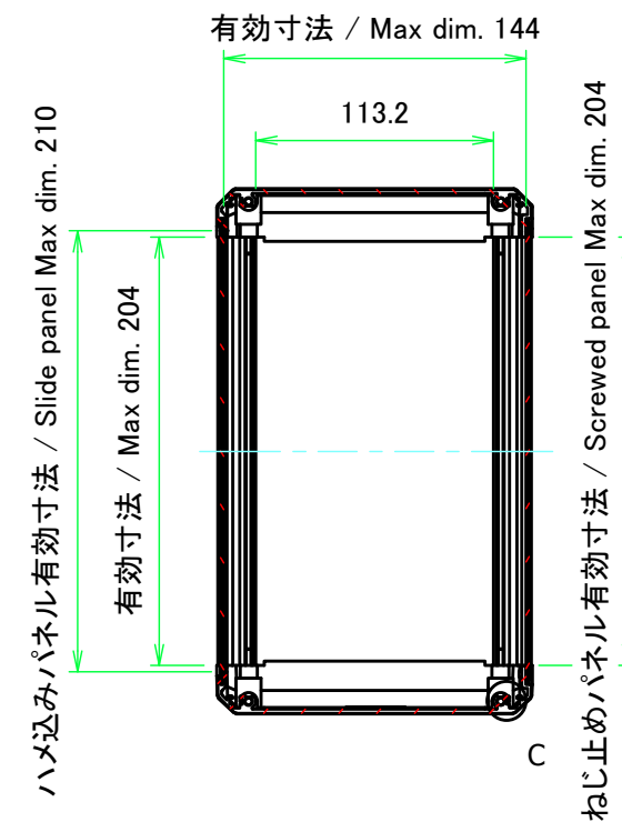
B-B ( 1 : 4 )
